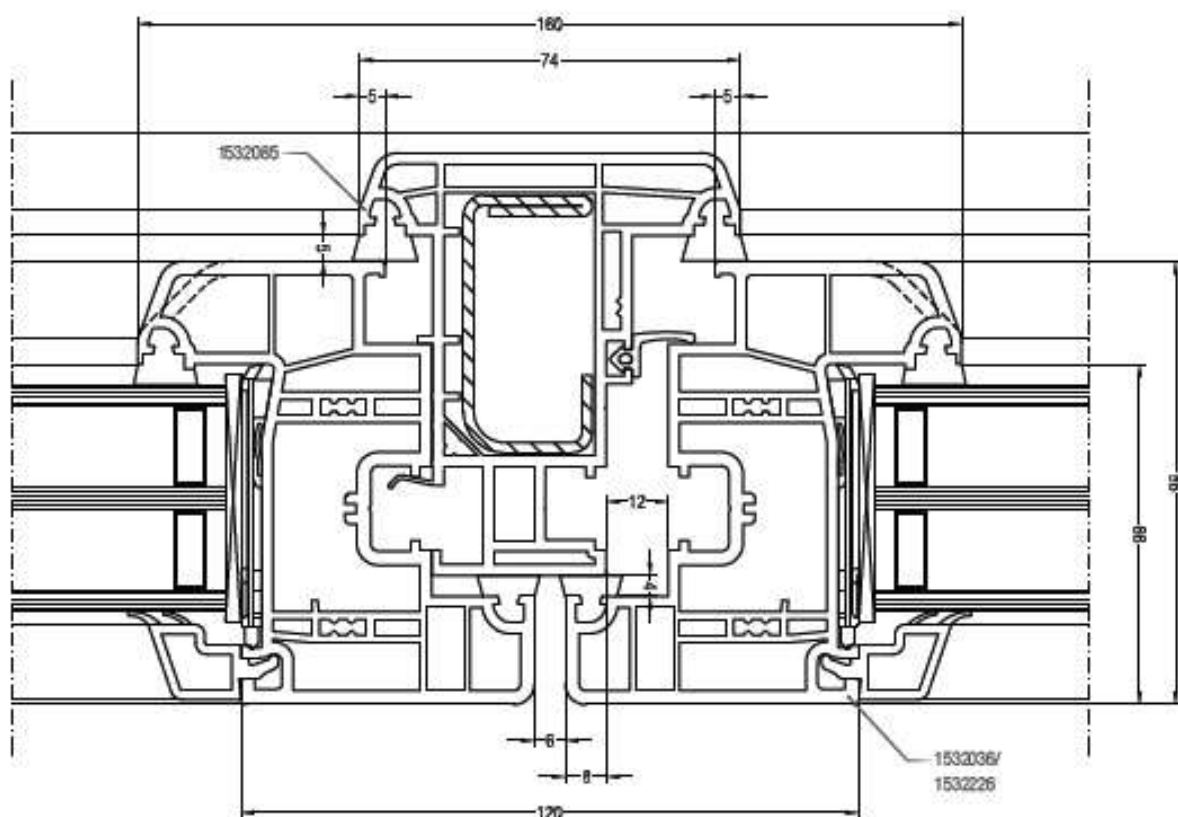
Sezione anta dritta da 57 mm - 2 ante
