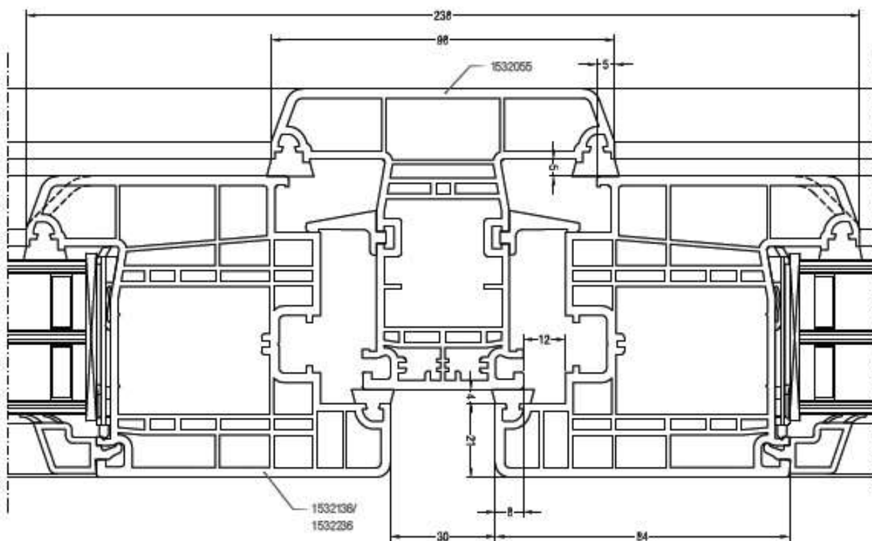
Sezione anta dritta da 84 mm - 2 ante
